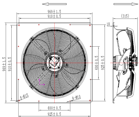
Рис. 1 - Габаритные размеры вентилятора
