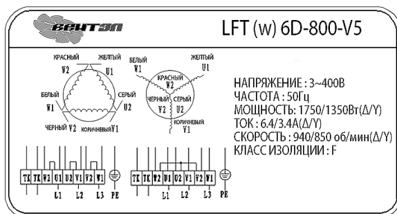
Рис. 2 - Схема подключения
