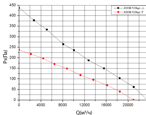
Рис. 3 - Кривая производительности
