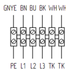
Схема №3 400В, 3ф, 50Гц
